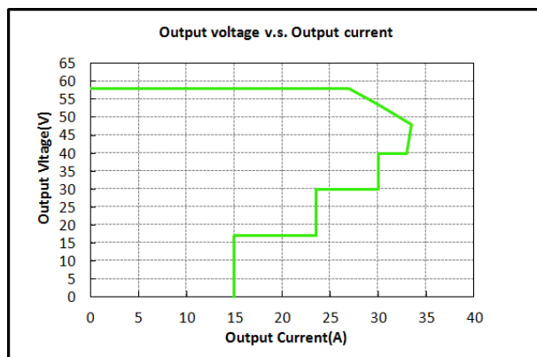
图1 输出外特性曲线图
