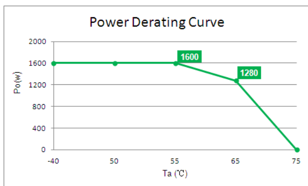
图3 R4830G1功率降额曲线
